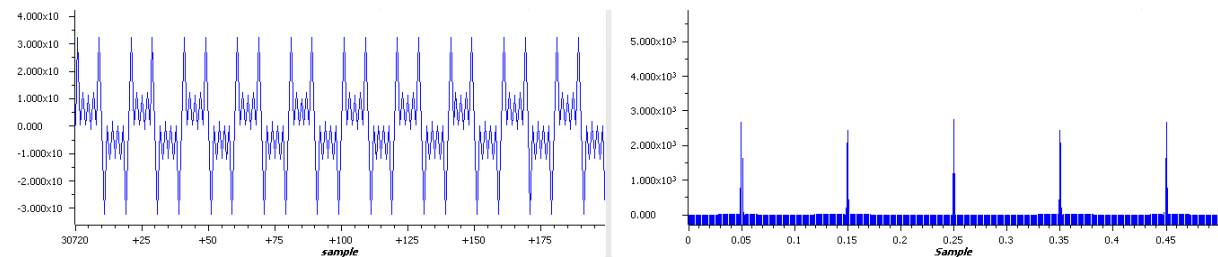
Slika 3 - Multiton signal za f_0=0.05 , df=0.1 prikazan u vremenskom i frekventnom domenu
